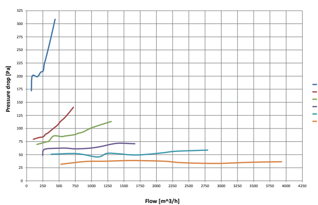
Nyomásdiagramm DAOSL-K
