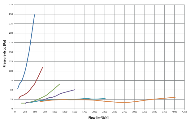
Nyomásdiagramm DAOSL
