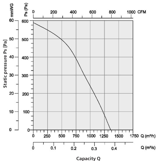
Fan flow curves DV-355
