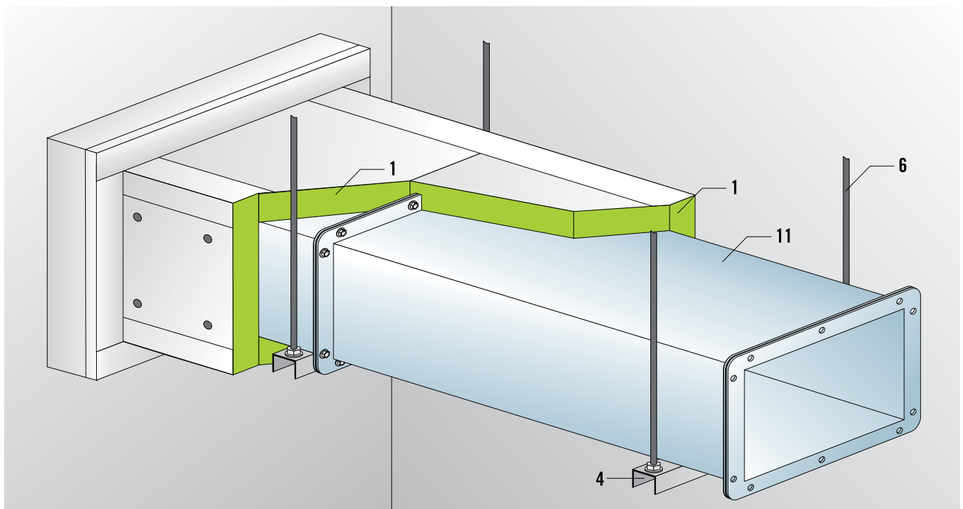
Ábra: 1. CONLIT Ductrock / CONLIT Plus; 4. U-alakú fémfelfüggesztés; 6. Fémpálca; 11. Szellőzőcsatorna
