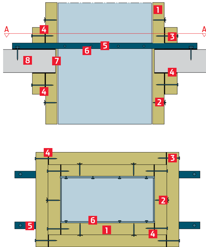
A földemen átmenő csatorna keresztmetszete
