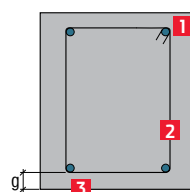
II/1. ábra. Vasbeton gerendák és oszlopok 1. vízszintes vasbeton gerenda, 2. betonacél, fő vasalás, 3. „g” fő vasalás betonfedése
