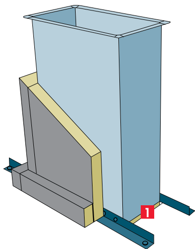
A földémen átvezetett csatorna nézete
