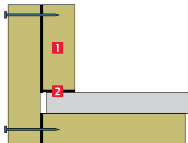
I/4. ábra: 1. A toldólemez külső síkja a szerkezeti acélelem oldalsó élén kívül legyen. 2. CONLIT Glue ragasztó és az illesztési ragasztás biztosítása rögzítő szegekkel.
