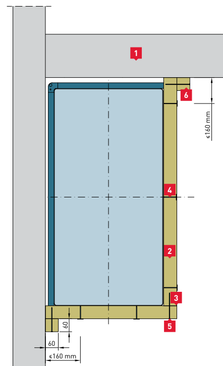
Függőleges csatorna 2-oldali szigetelése
