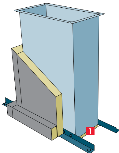
A födémén átvezetett csatorna nézete 1. A nyílás kőzetgyapattal való kitöltése
