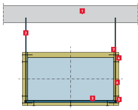
Vízszintes csatorna 2-oldali szigetelése.
