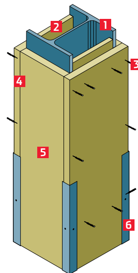
I/11. ábra. Az oszlop négyoldalas beépítése
