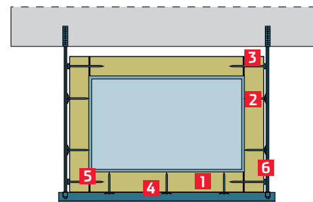
Csatorna a felfüggesztéssel a szigetelésen kívül
