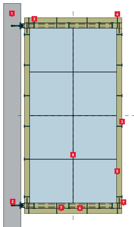
Függőleges csatorna 4-oldali szigetelése
