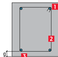
II/1. ábra. Vasbeton gerendák és oszlopok 1. vízszintes vasbeton gerenda, 2. betonacél, fő vasalás, 3. „g” fő vasalás betonfedése
