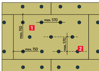
II/4. ábra. Mechanikai rögzítés elhelyezése
