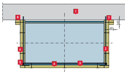
Vízszintes csatorna 4-oldali szigetelése
