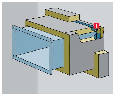
A csatornát merevítő acél szögvas szerelési módja a CONLIT Ductrock / Plus lemez esetében.
