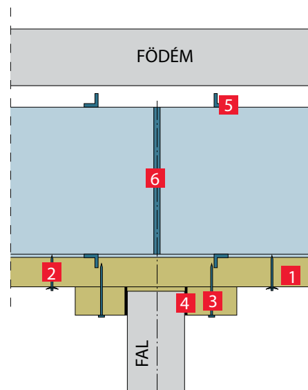
Két- vagy háromoldalúan szigetelt vezeték a falon keresztül való átvezetése
