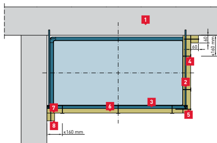
Vízszintes csatorna 3-oldali szigetelése
