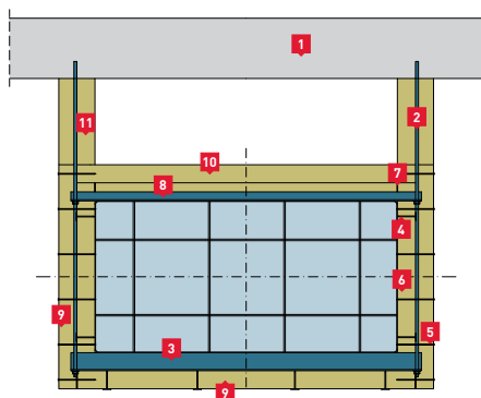
Függőleges csatorna 4-oldali szigetelése
