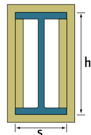
I/3. ábra: A CONLIT 150 tűzvédelmi burkolat leggyakoribb beépítési formája a dobozos védelem
