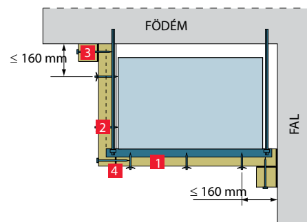
CONLIT Ductrock / Plus lemezekkel kétoldalúan szigetelt vízszintes csatorna.
