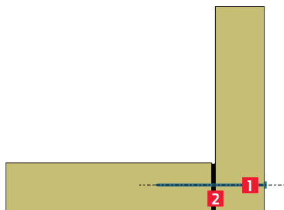
I/1. ábra: Sarok illesztések egyszerű ragasztással
