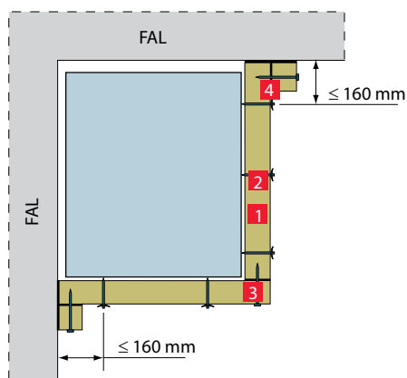
CONLIT Ductrock / Plus lemezekkel kétoldali szigetelt függőleges csatorna
