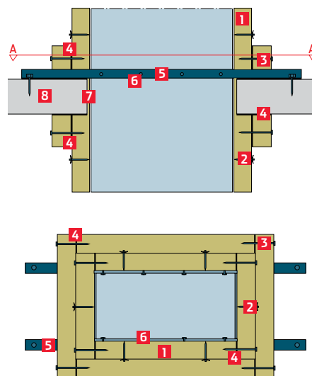
A födémén átmenő csatorna keresztmetszete 1. CONLIT Ductrock/Plus, 2. acél túske, 3. szerelési szeg, 4. CONLIT Glue ragasztó, 5. 50 x 50 x 5,0 mm-es acél szög, 6. menetes csavarok, 7. ömlesztett kőzetgyapot, 8. emeletek közötti födém
