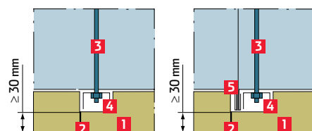
A csatorna felfüggesztésének szigetelése
